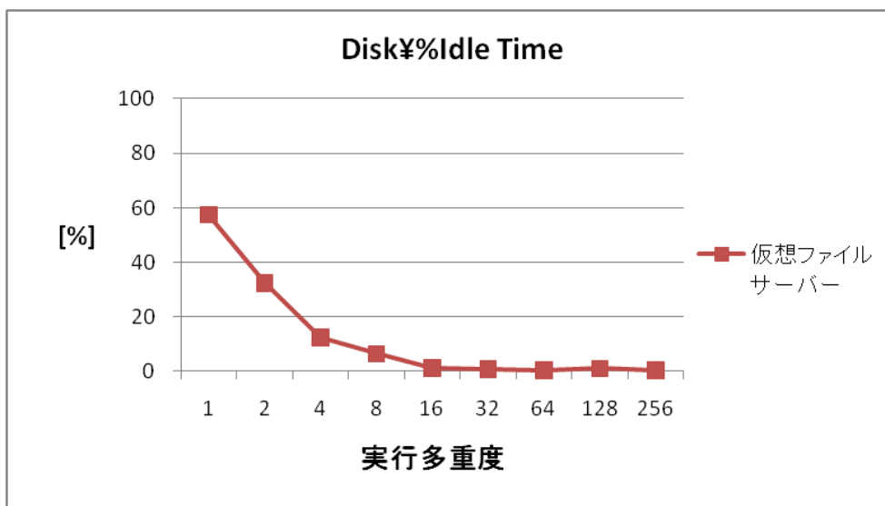
図 6-9 仮想ファイルサーバー Disk %Idle Time
