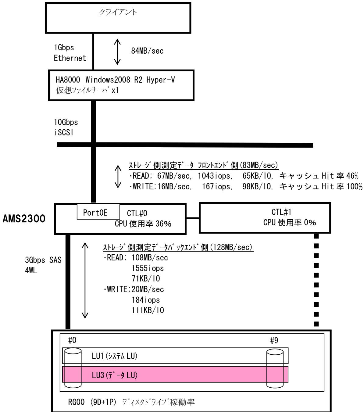
図 6-15 多重度 128 における AMS2300 の稼働状態
