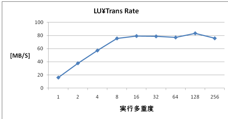
図 6-12 ディスク転送量
