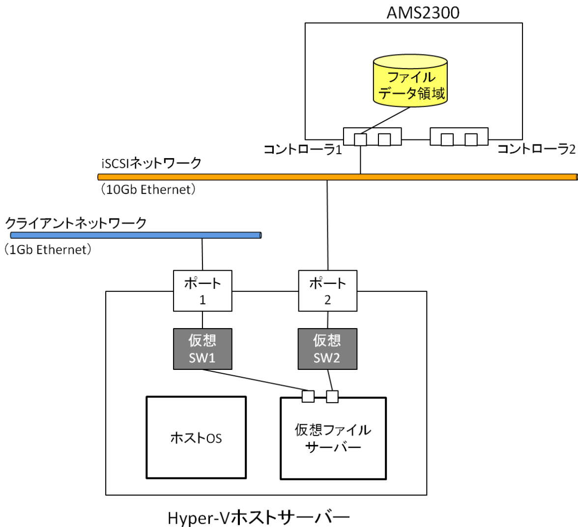
図 4-2 仮想ファイルサーバー構成図
