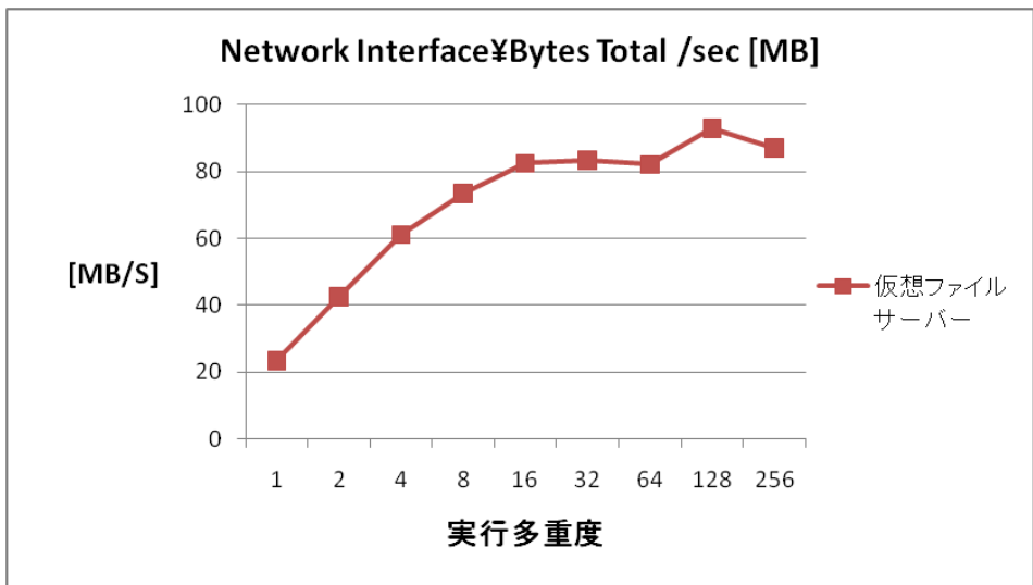
図 6-7 仮想ファイルサーバー ネットワーク転送量
