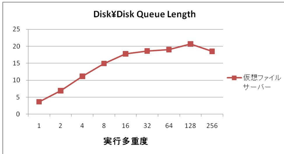
図 6-10 仮想ファイルサーバー Disk¥Avg.Disk Queue Length
