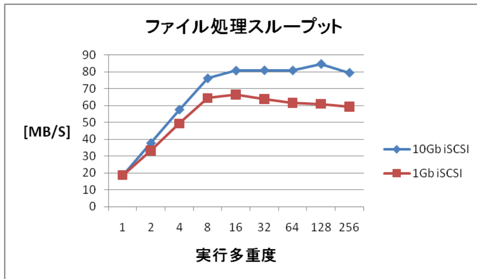
図 7-7-1 10Gb iSCSI 構成と 1Gb iSCSI 構成のファイル処理スループットの比較
