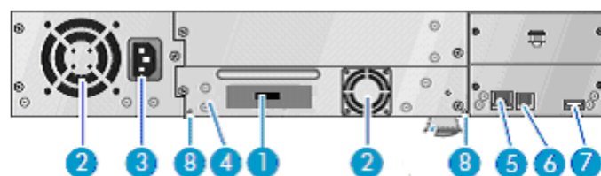
装置背面図
