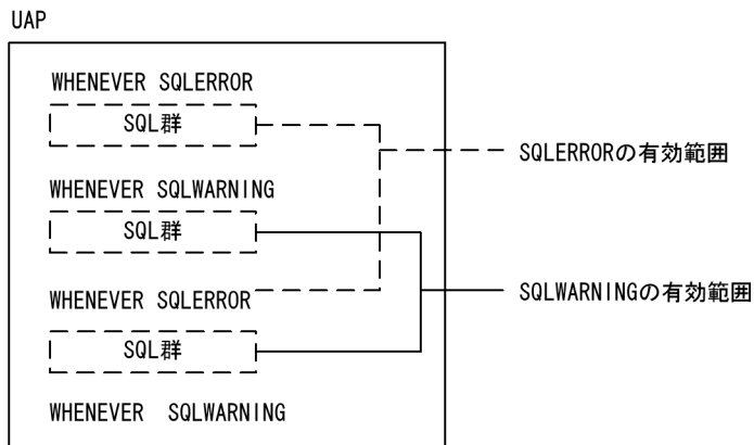
図 6-1 埋込み例外宣言で指定した処理の有効範囲
