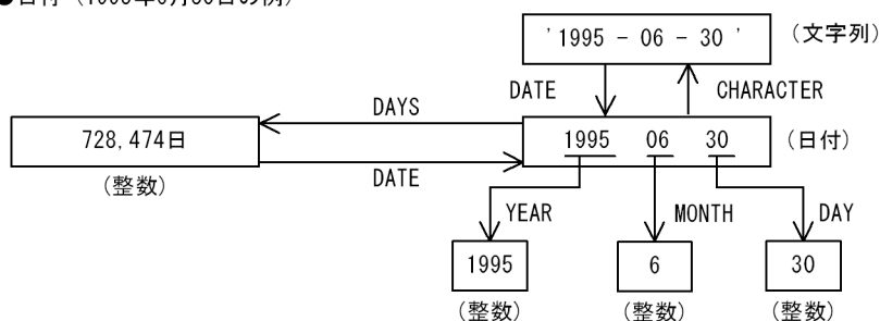
図 2-6 日付データ、時刻データ、時刻印データ、及び数データへのシステム組込みスカラ関数の実行例
