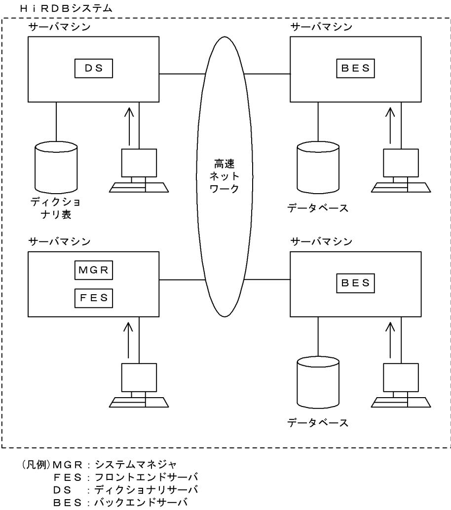
図 1-2 コマンドの実行形態（HiRDB/パラレルサーバの場合）
