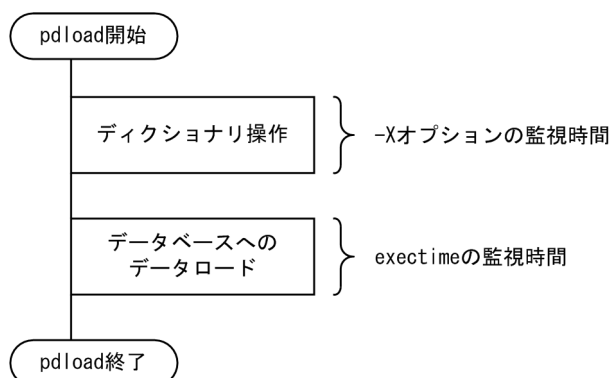
図 5-14 pload 実行時の監視時間範囲の関係
