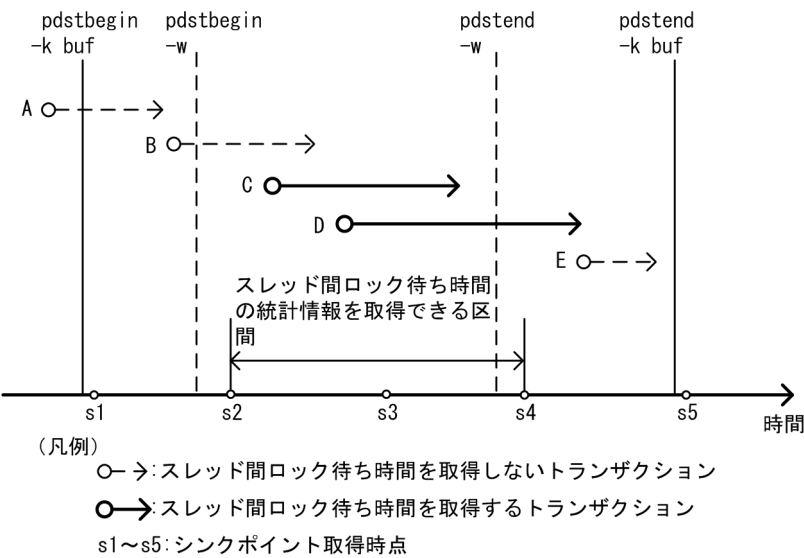
図 2-11 スレッド間ロック待ち時間の統計情報を取得できる区間 (buf)
