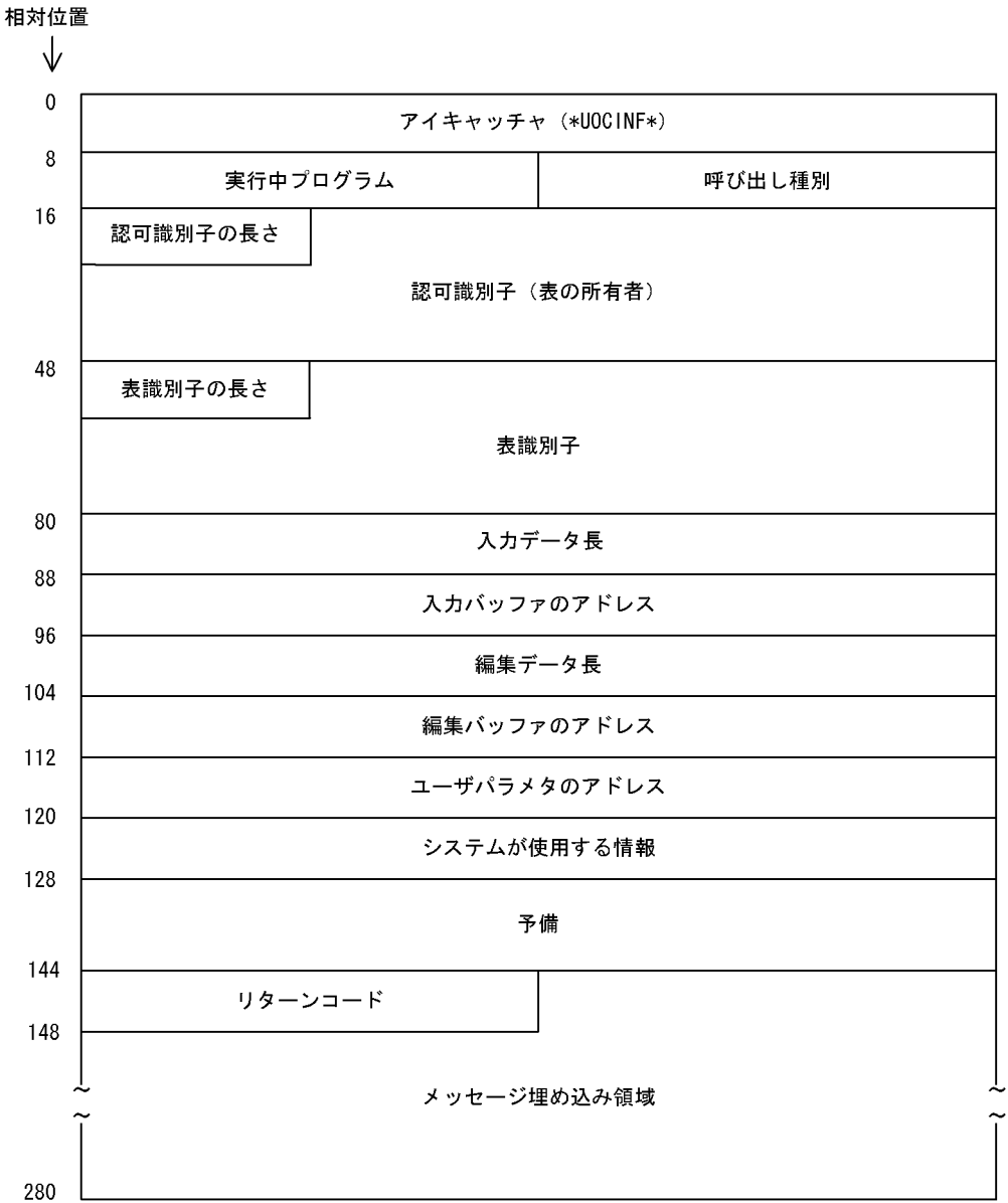
図 5-31 UOC インタフェース領域の構造 (64 ビットモードの場合)
