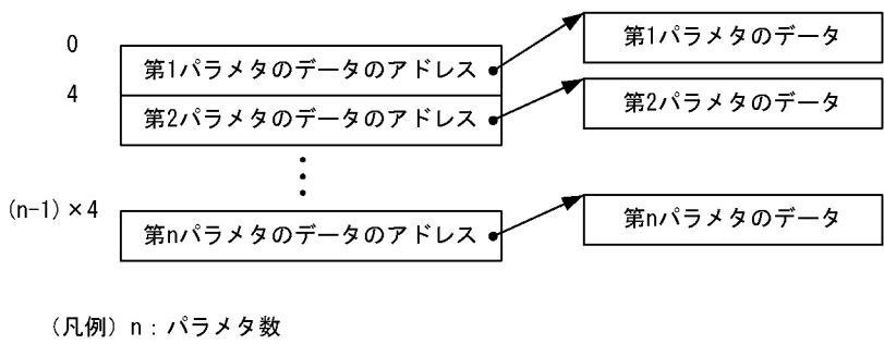
図 8-30 抽象データ型パラメタのアドレスリストの構造
