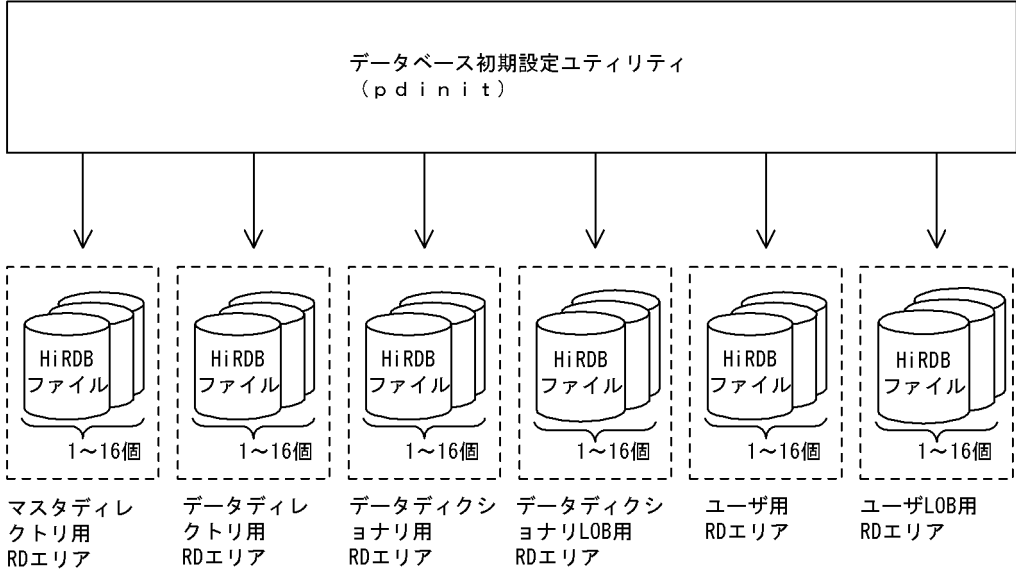
図 3-1 データベース初期設定ユーティリティ (pdinit) の概要
