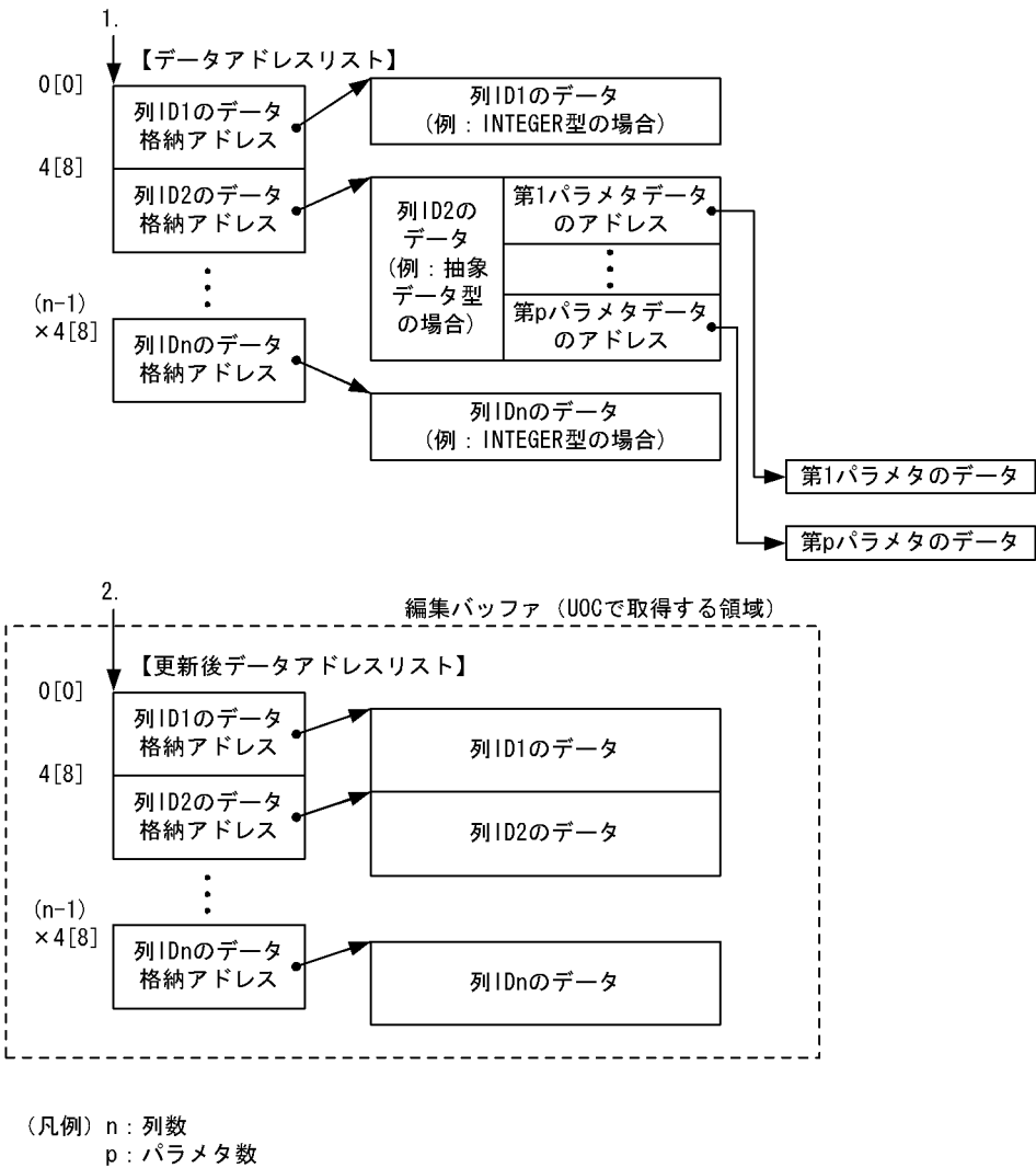
図 8-29 UOC インタフェース領域の構造 (2/2)
