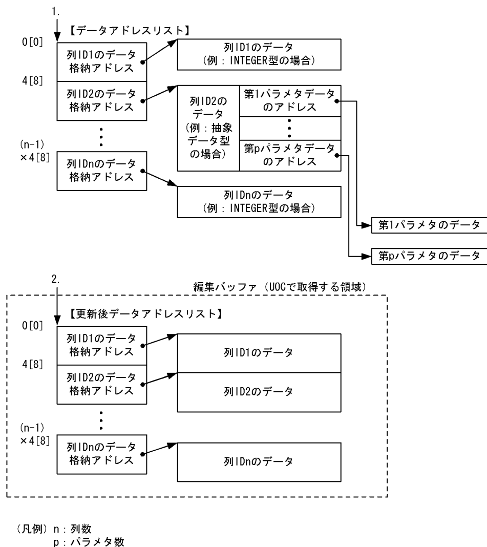
図 8-30 UOC インタフェース領域の構造 (2/2)
