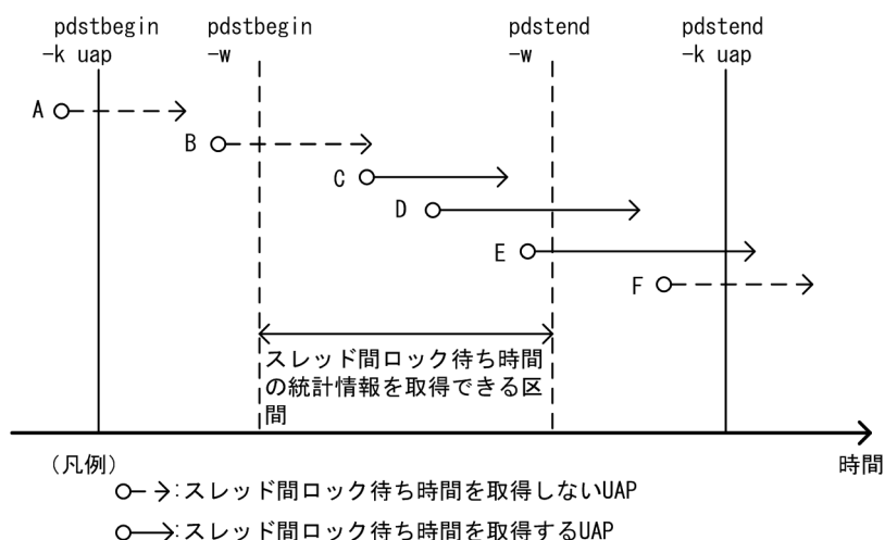
図 2-17 スレッド間ロック待ち時間の統計情報を取得できる区間 (uap)
