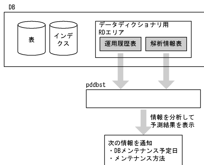
図 15-7 再編成時期予測機能の概要
