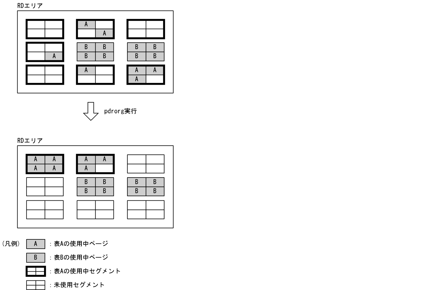
図 11-6 pdrorg を実行した場合の使用中空きページ，及び使用中空きセグメントの解放
