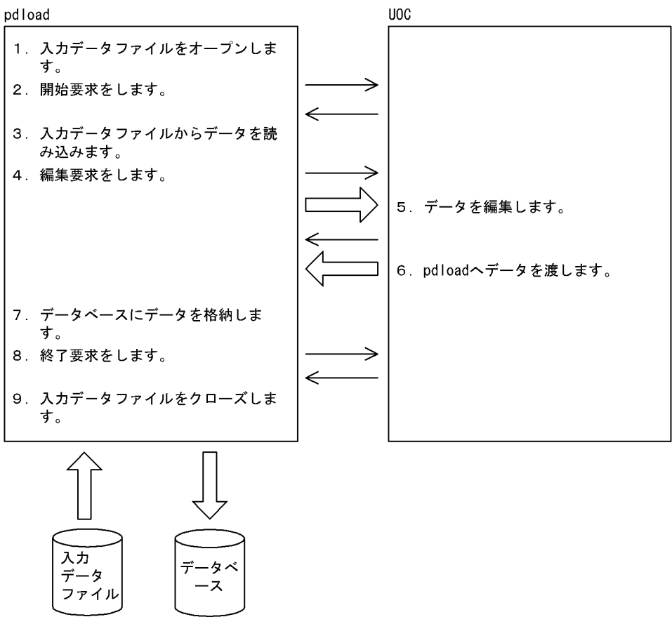
図 5-29 UOC を利用した場合の表の作成方法 (ユティリティが入力データファイルを入力する方法)
