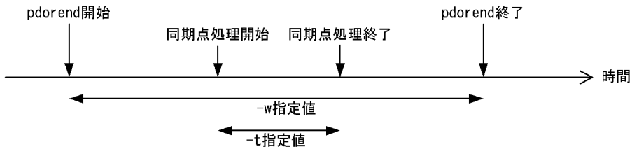
図 2-12 追い付き反映処理の最大待ち時間、及びトランザクション処理の最大待ち時間の関係
