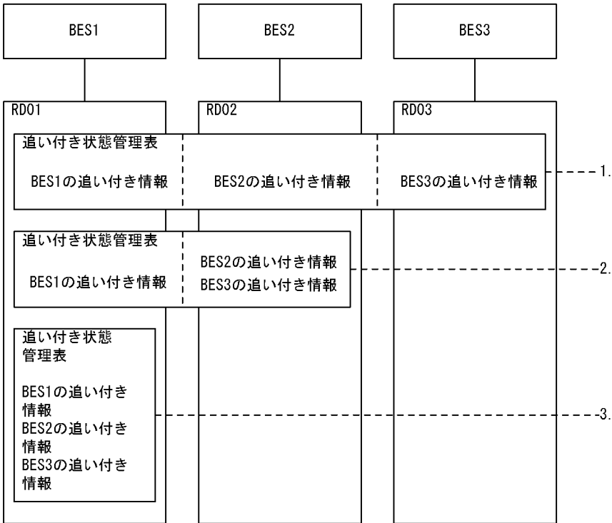
図 2-8 BES1, BES2, 及び BES3 に追いつき状態管理表を作成する例
