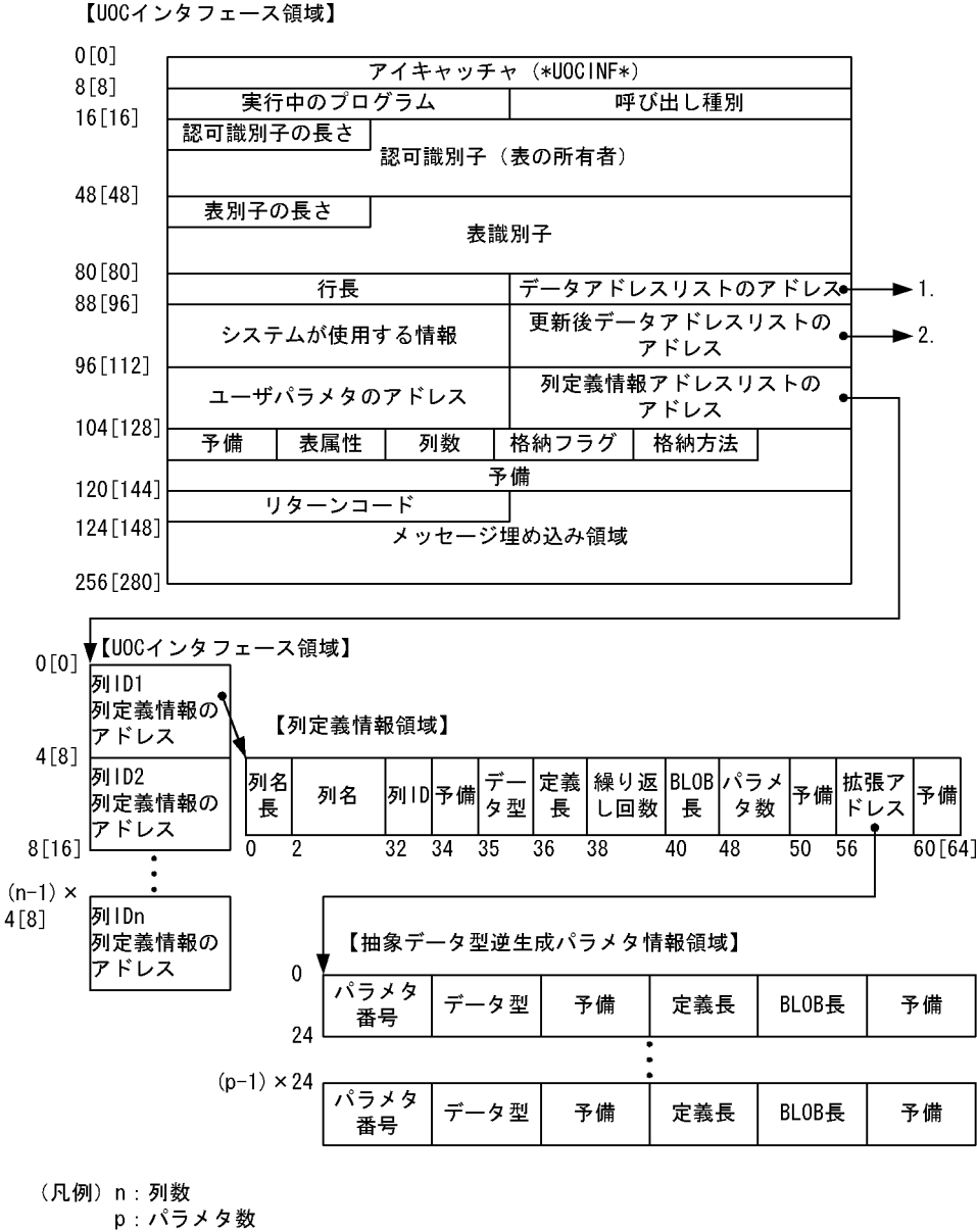
図 8-29 UOC インタフェース領域の構造 (1/2)
