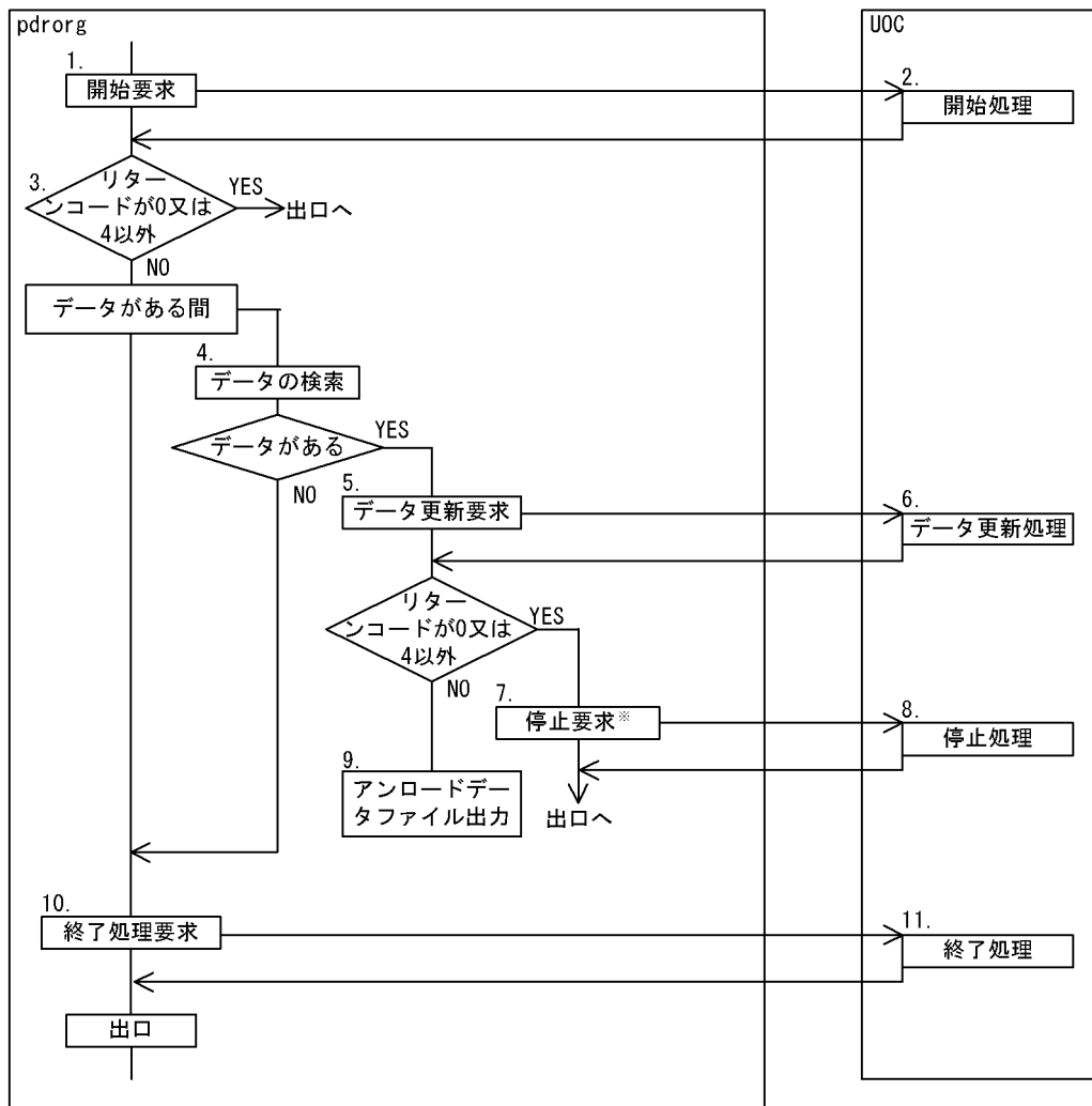
図 8-28 pdrorg, UOC 間の呼び出しシーケンス
