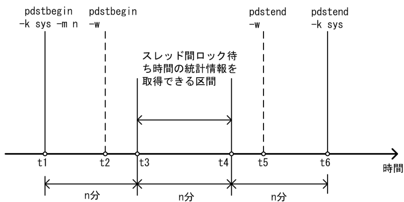
図 2-16 スレッド間ロック待ち時間の統計情報を取得できる区間 (sys)
