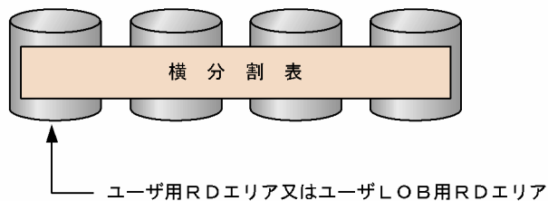
図 3-8 表の横分割
