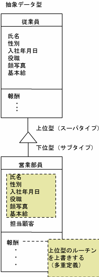
図 3-42 多重定義
