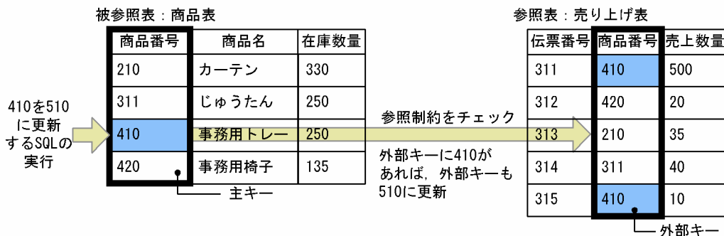
図 5-9 被参照表に更新 SQL を実行するときの動作の例（CASCADE 指定時）
