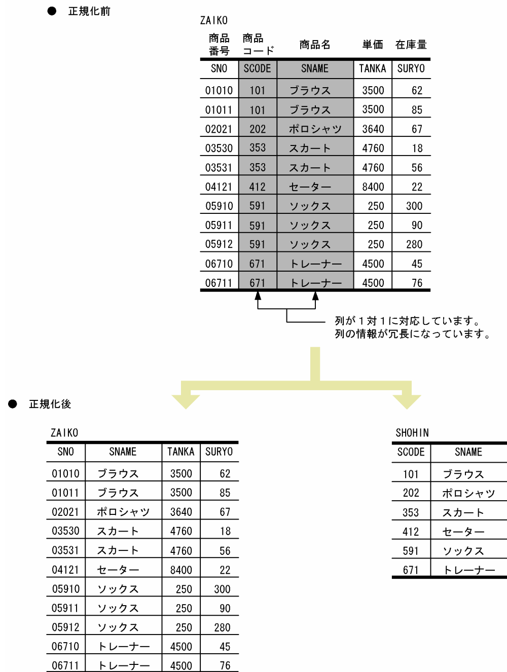
図 3-5 表の正規化
