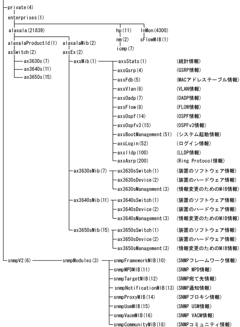
図 1-2 MIB 体系図 (2/2)
