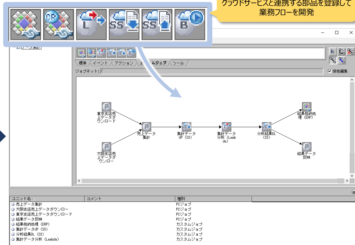
ジョブネットエディタ画面
