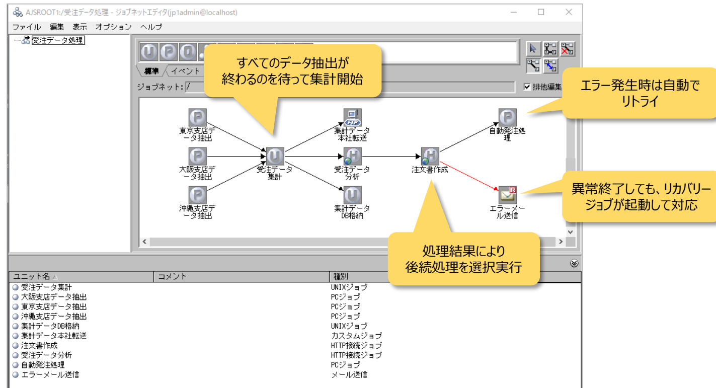
ジョブネットエディタ画面
