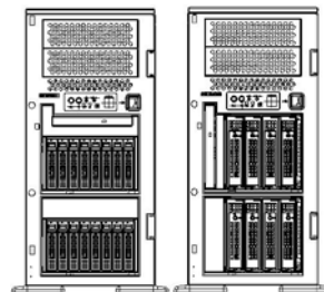
標準モデル
