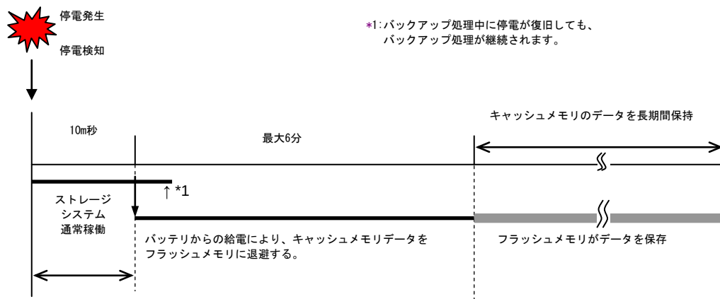
停電時のキャッシュメモリのバックアップ動作
