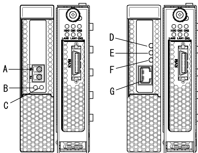
サーバモジュール+ライザーカード+ Fibre Channel ボード
