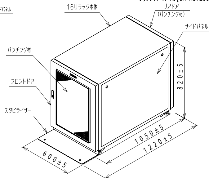
(2) ラックキャビネット (16U) [GH-RK7166] + フロントドア [GH-RD7167] + リアドア [GH-RD7168] + ラックサイドパネル [GH-RS7166]
