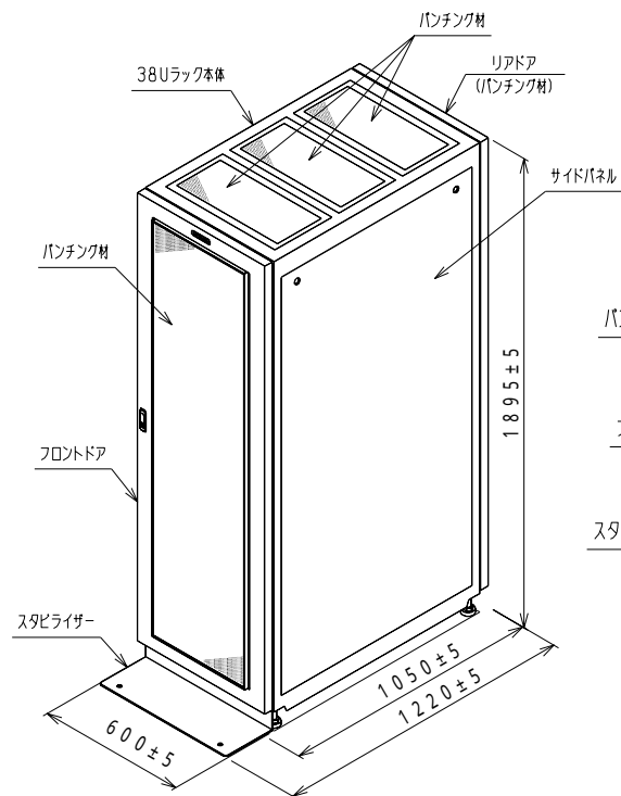
(1) ラックキャビネット (38U) [GH-RK7386] + フロントドア [GH-RD7386] + ラックサイドパネル [GH-RS7386]
