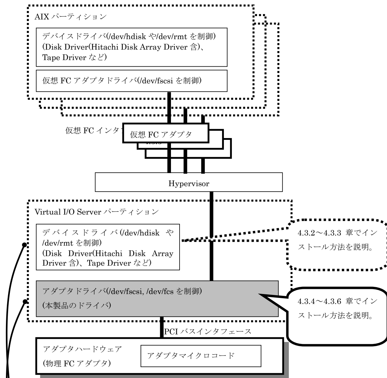
図 4-3-1 Virtual I/O Server パーティションに搭載されたアダプタハードウェア
