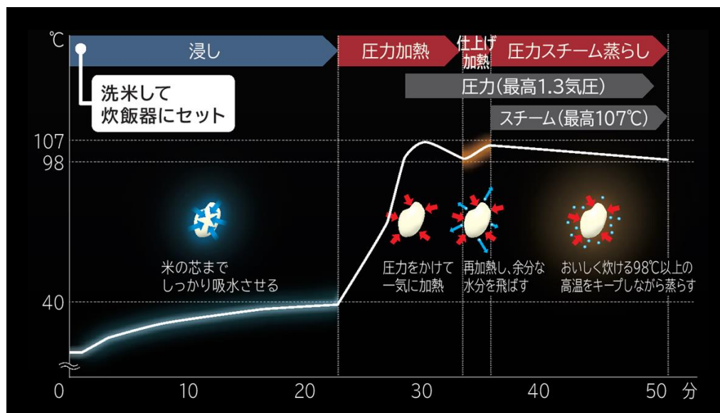
[図 2 極上ひと粒炊きの炊飯工程]
