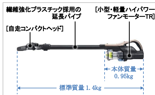
[図1 質量と軽量化のポイント]
