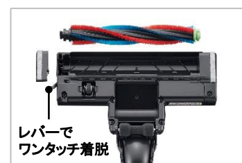
[図5 ワンタッチ着脱]
