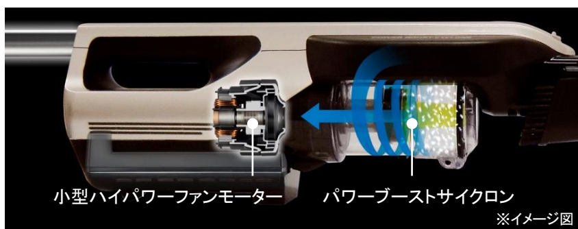
【図4 小型ハイパワーファンモーターとパワーブーストサイクロン】
