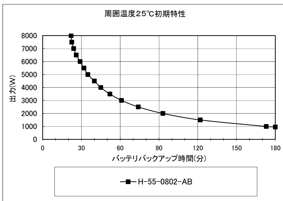
図9. 1 バッテリバックアップ時間
