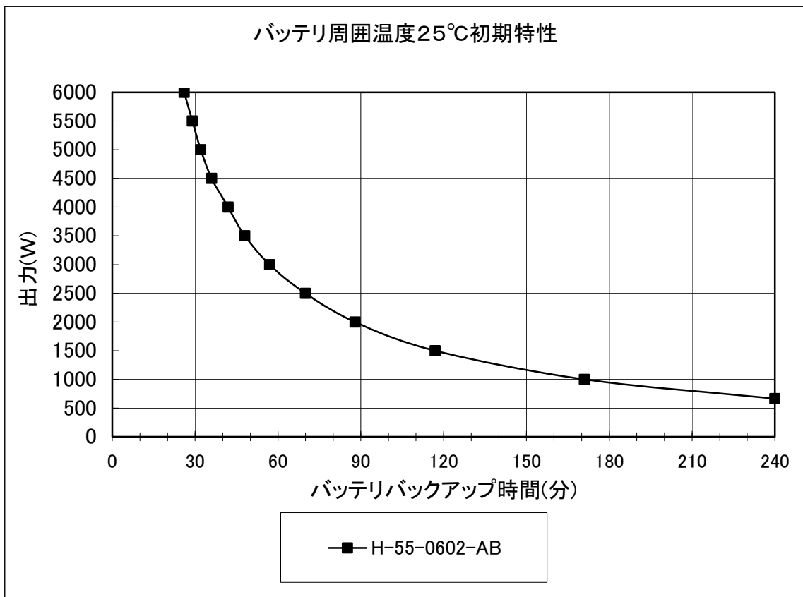
図9. 1 バッテリバックアップ時間
