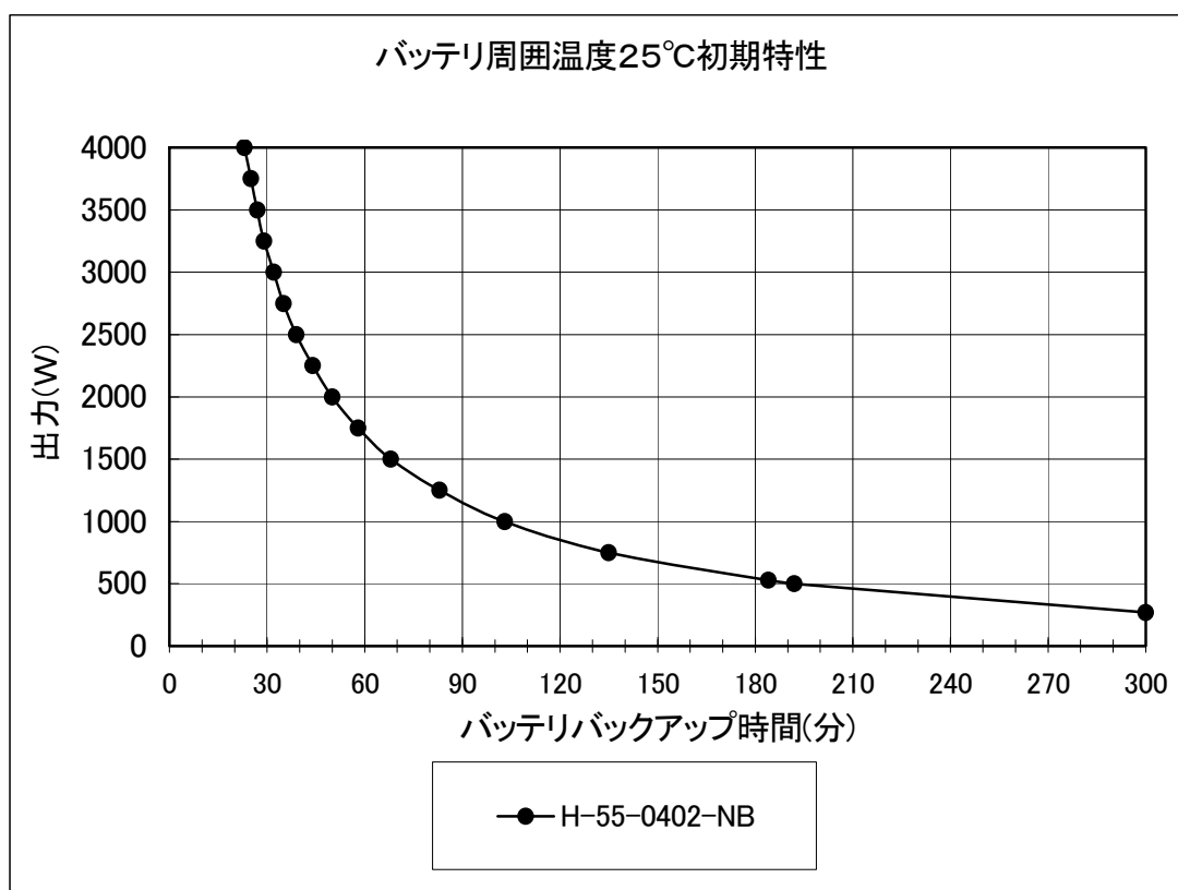
図9. 1 バッテリバックアップ時間
