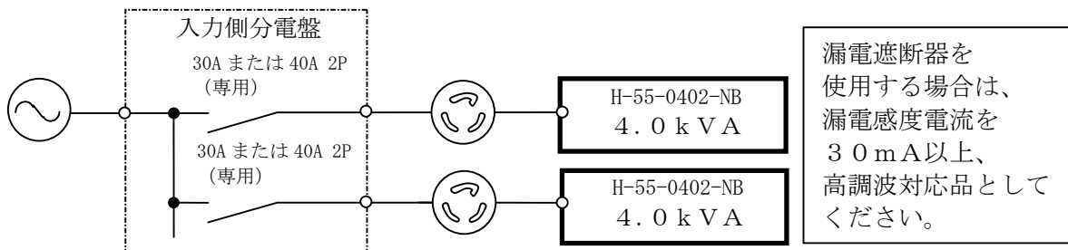
図 3. 1 電源接続図
