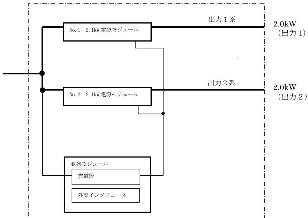
図 6. 4 2 系統電源の構成
