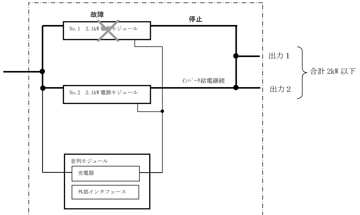
図 6. 3 冗長電源の動作例
