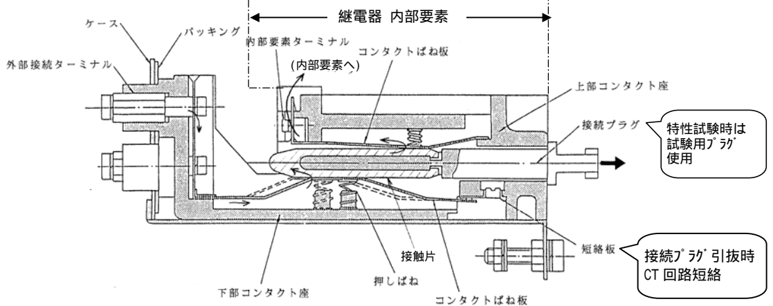
引出形継電器のプラグ機構
