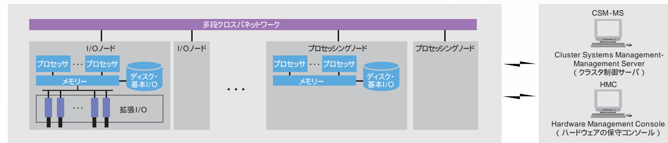
SR11000 モデルH1のシステム構成
