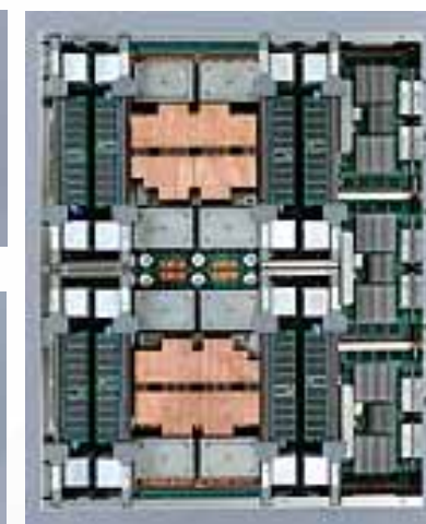
1ノードを搭載したパッケージ
