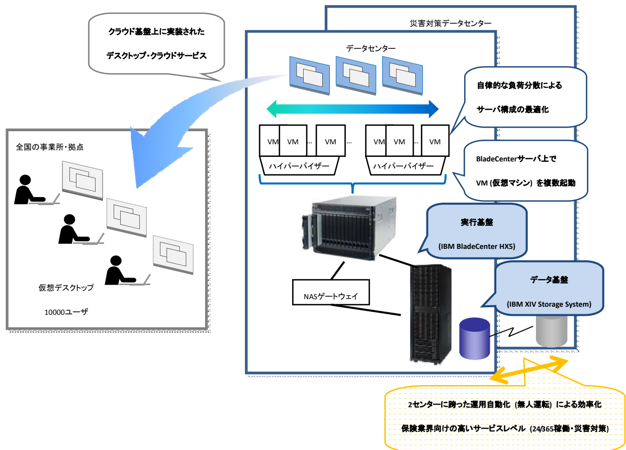
添付図 1: NISSAY IT 保険業界向けクラウド基盤 システム構成イメージ図
