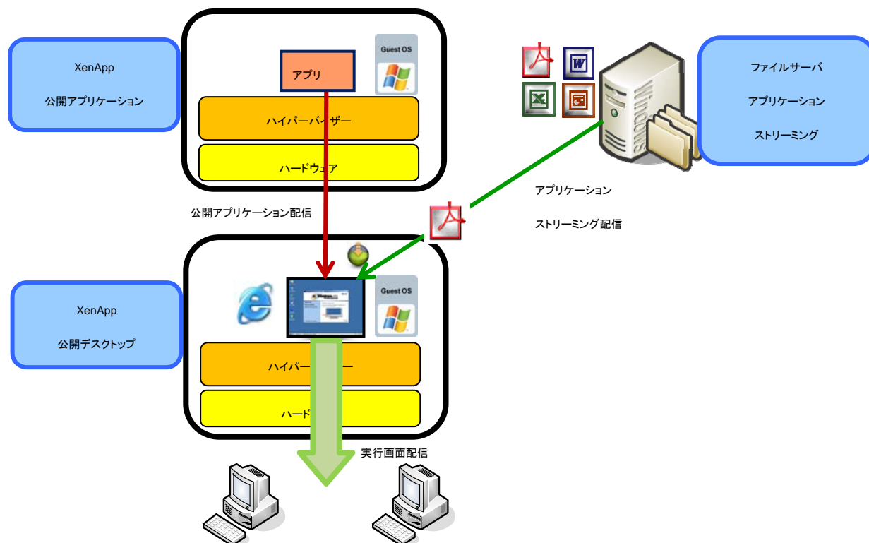
添付図 2: アプリケーション仮想化 構成イメージ図
